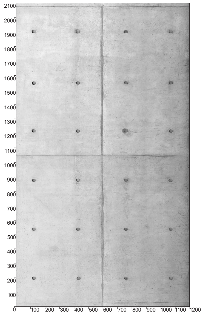
Betonwand mit Fugen senkrecht zu 1200 mm Breite
